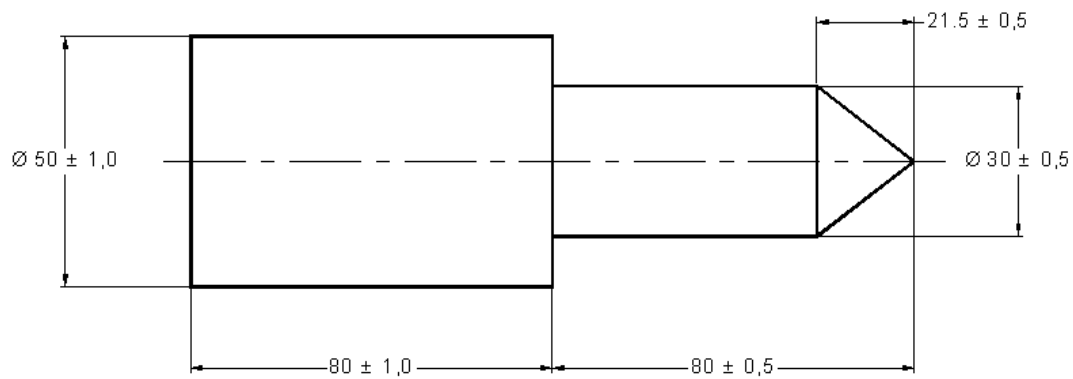
Figura 4. Probeta de prueba
