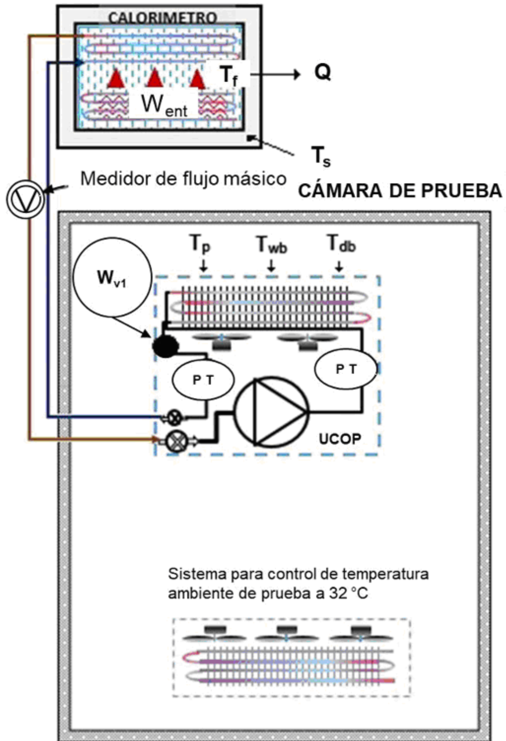
Figura 5 - Método calorímetro
